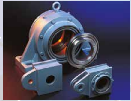
Soportes no partidos, material acero, para aplicaciones con altas cargas
